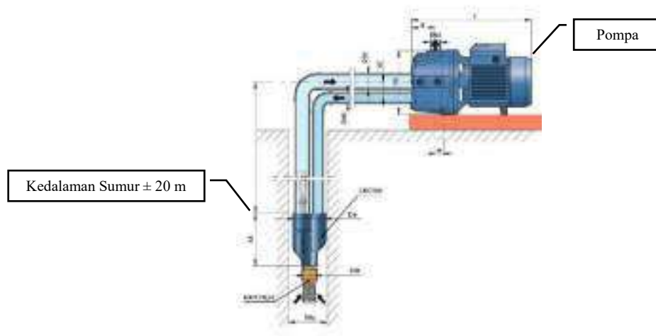
Gambar 3.2. Sketsa sumur bor dan pompa
