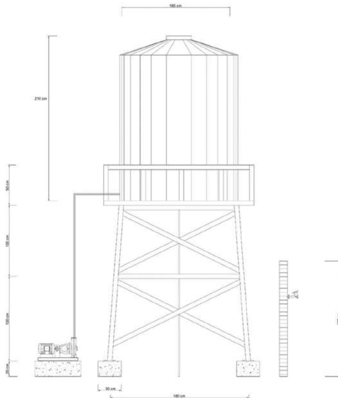
Gambar 2.1. Sumur Bor Beserta Tangki Air
