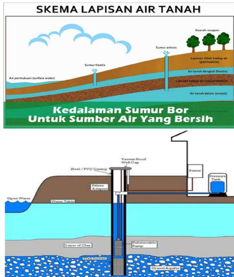
Gambar 2.2. Kedalaman Sumur Bor
